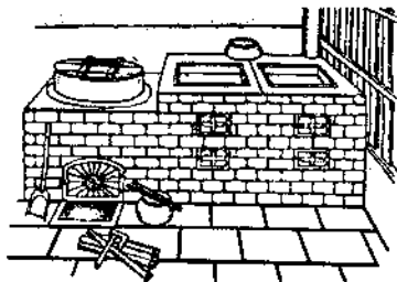
Hình 85: Lò chiên đậu và nấu đậu
