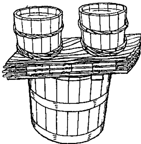
Hình 100: Cách ép đậu để chiên giòn
